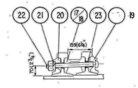
HEEL BLOCK ASSEMBLY
