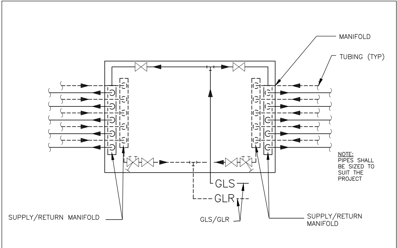
1 NEW MANIFOLD PIT PIPING M-405 SCALE : N.T.S.
